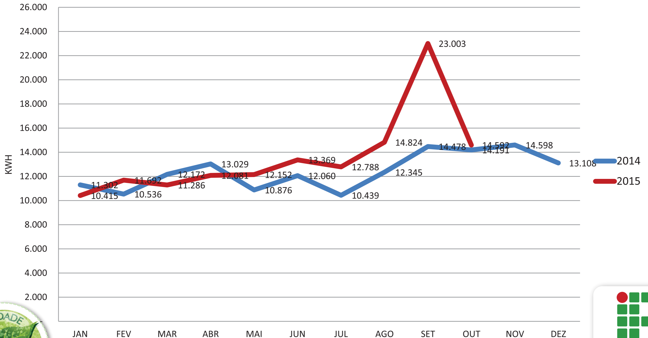
EVOLUÇÃO DO CONSUMO DE ENERGIA ELÉTRICA NA REITORIA/IFRO (em KWH) 2014 x 2015
